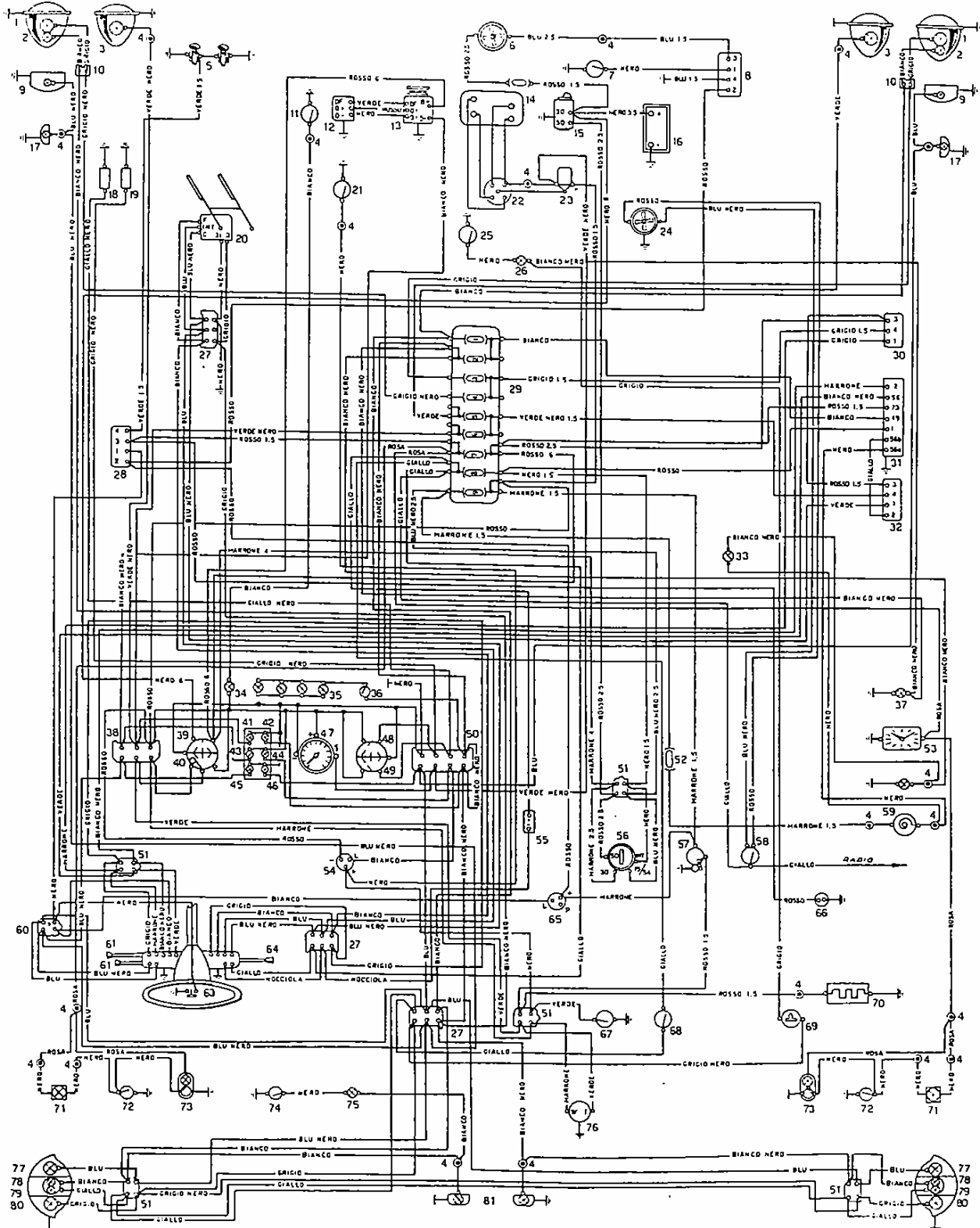
Schéma installation électrique berline (818.612).
