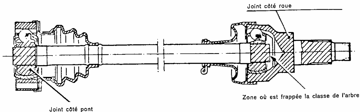
Fig. 20. - Arbre de roue avec ses joints.
