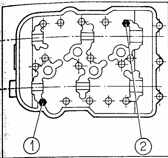
Fig. 7. - Position de montage des vis-ergots pour le centrage de la culasse.
