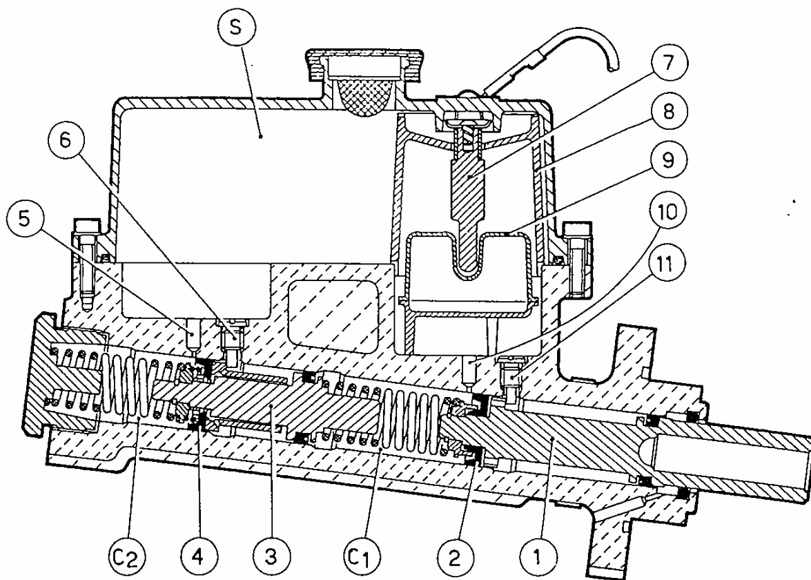
Fig. 27. - Maître-cylindre freins.
