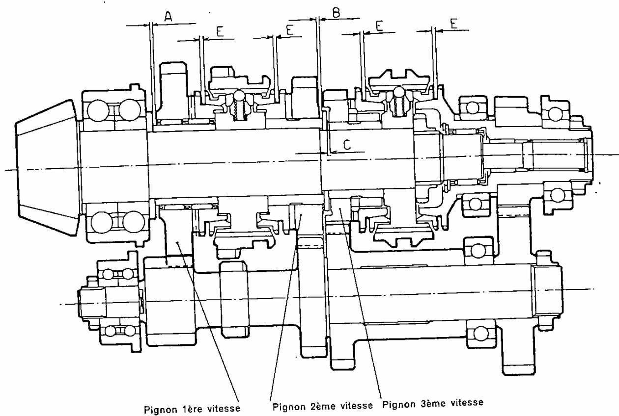
Fig. 15. - Pignonerie boîte à 4 vitesses.
