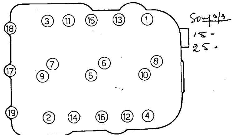
Fig. 8. - Ordre de serrage de la culasse.
