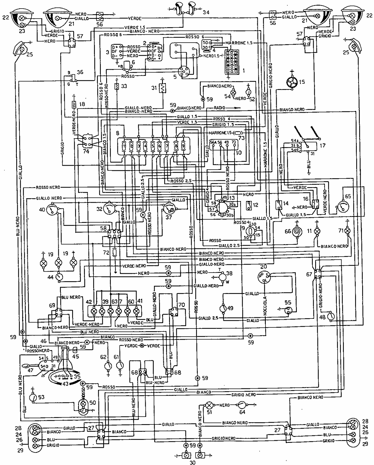
Schéma installation électrique coupé rallye 1,6 HF (818.540).
