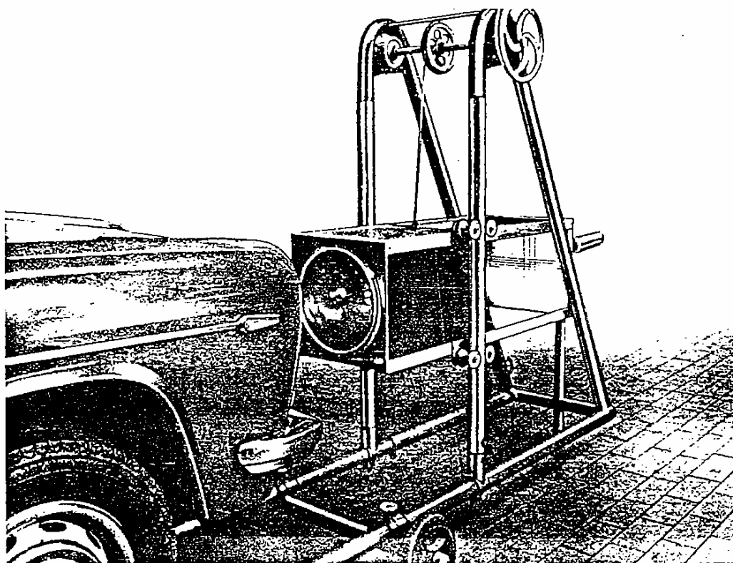
Fig. 33. - Contrôle des phares.
