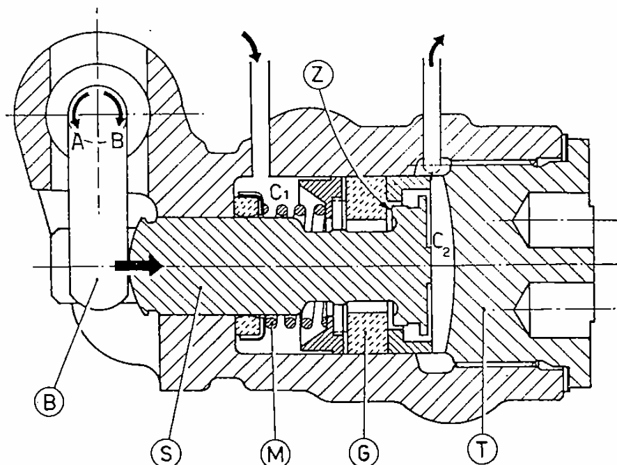
Fig. 29. - Régulateur de freinage.
