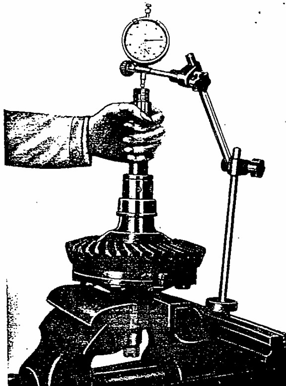
Fig. 19. - Contrôle jeu axial entre satellites et planétaires.
