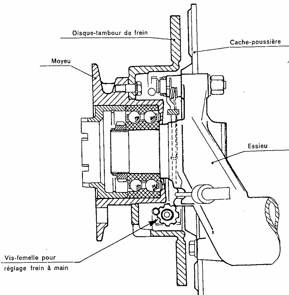
Fig. 31. - Coupe du disque de frein AR sur voiture.
