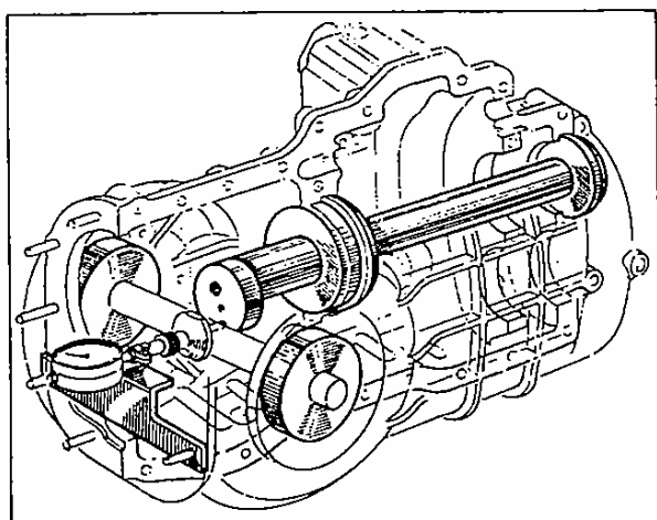
Fig. 17. - Réglage distance conique.
