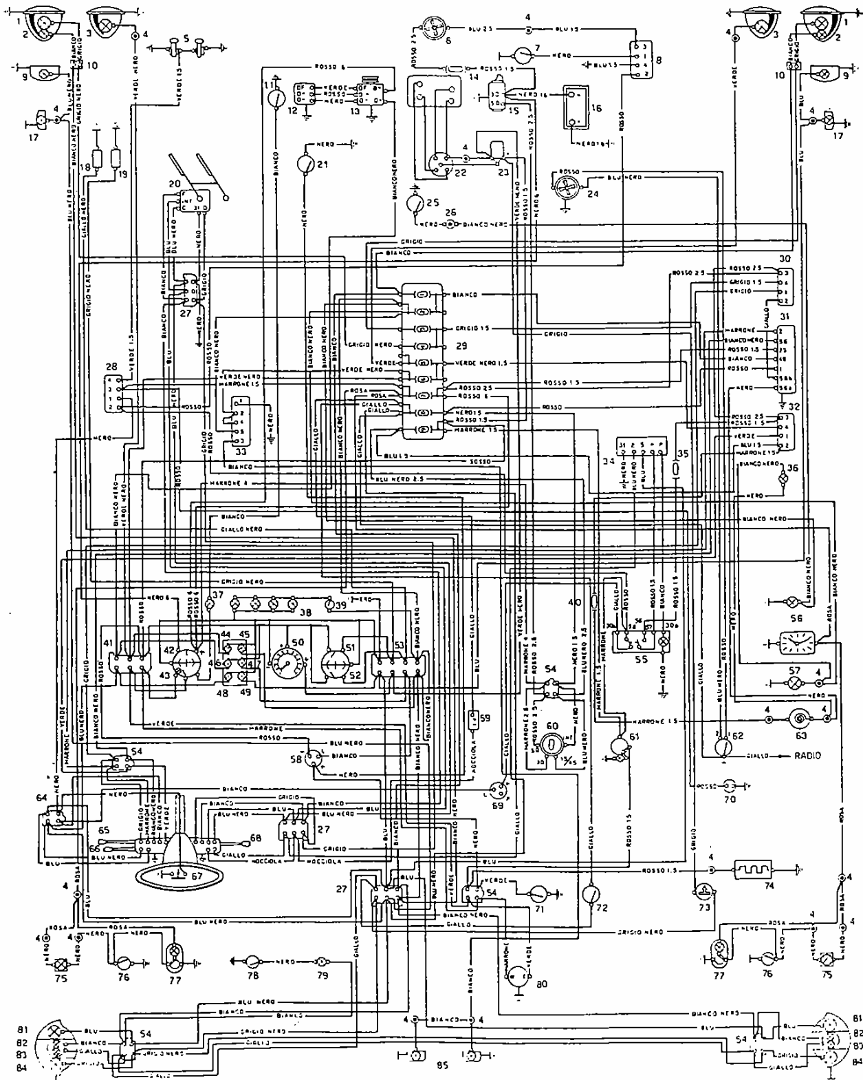
Schéma installation électrique berline (818.612) (pour voitures destinée dans ces Pays où est prévue l'application du signal de détresse).
