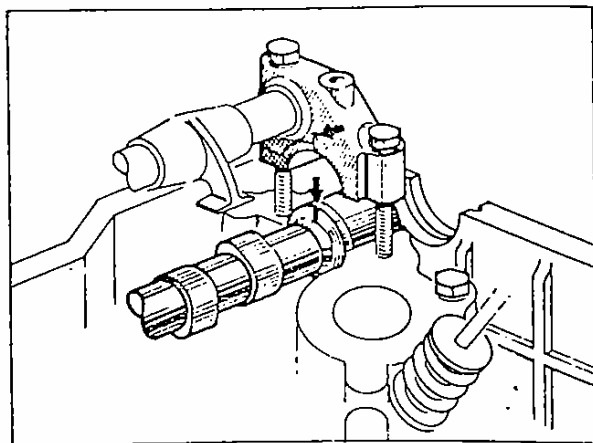
Fig. 11. - Position de montage arbres à cames.
