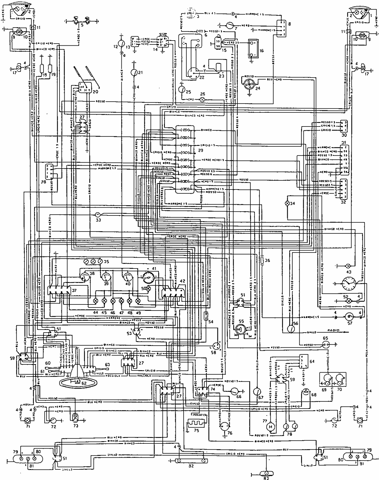
Schéma installation électrique Sport (818.650).
