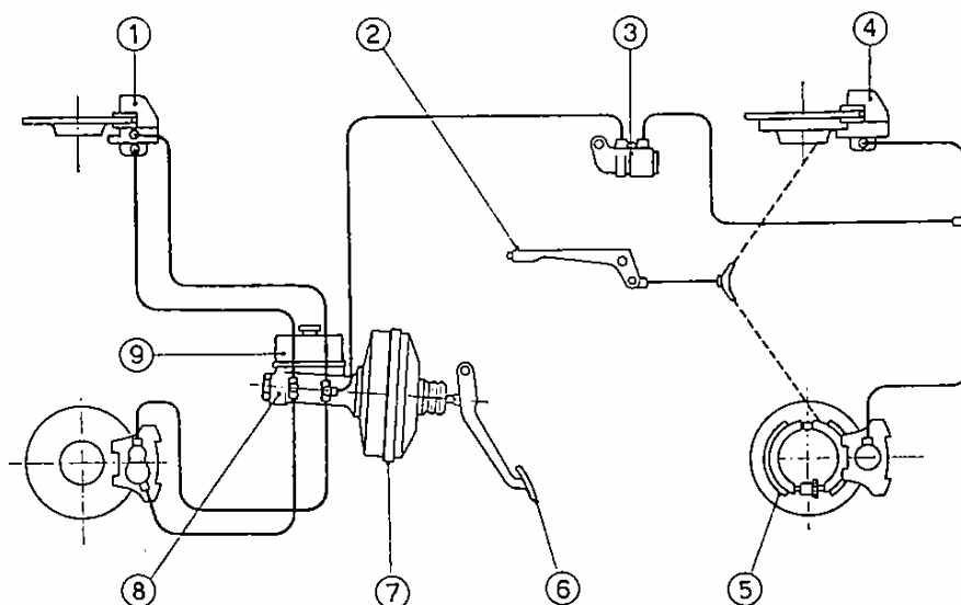
Fig. 25. - Système de freinage superduplex.
