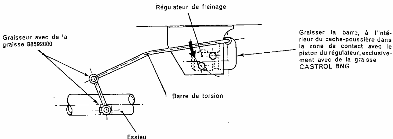
Fig. 30. - Mécanisme de commande du régulateur de freinage.
