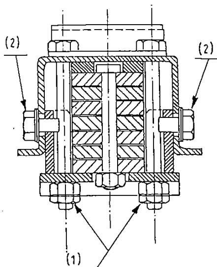
Fig. 24. - Coupe transversale du ressort à lames avant.
