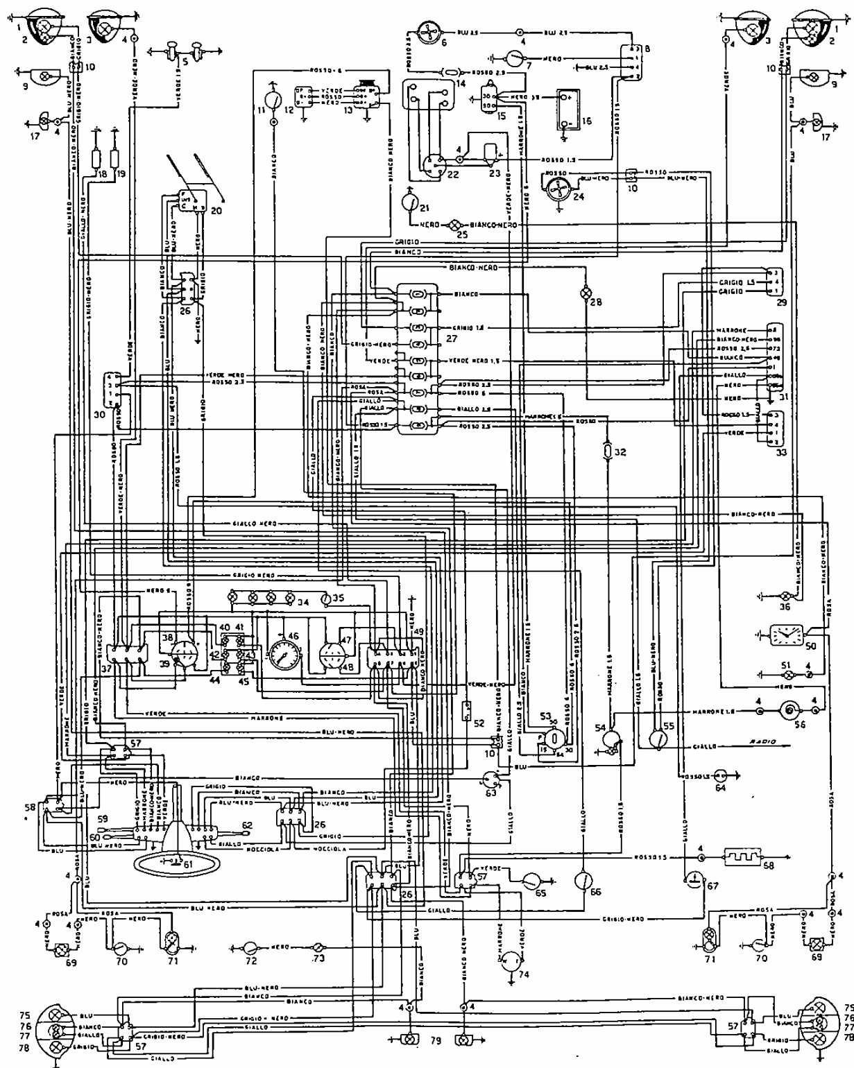
Schéma installation électrique berline (818.610).
