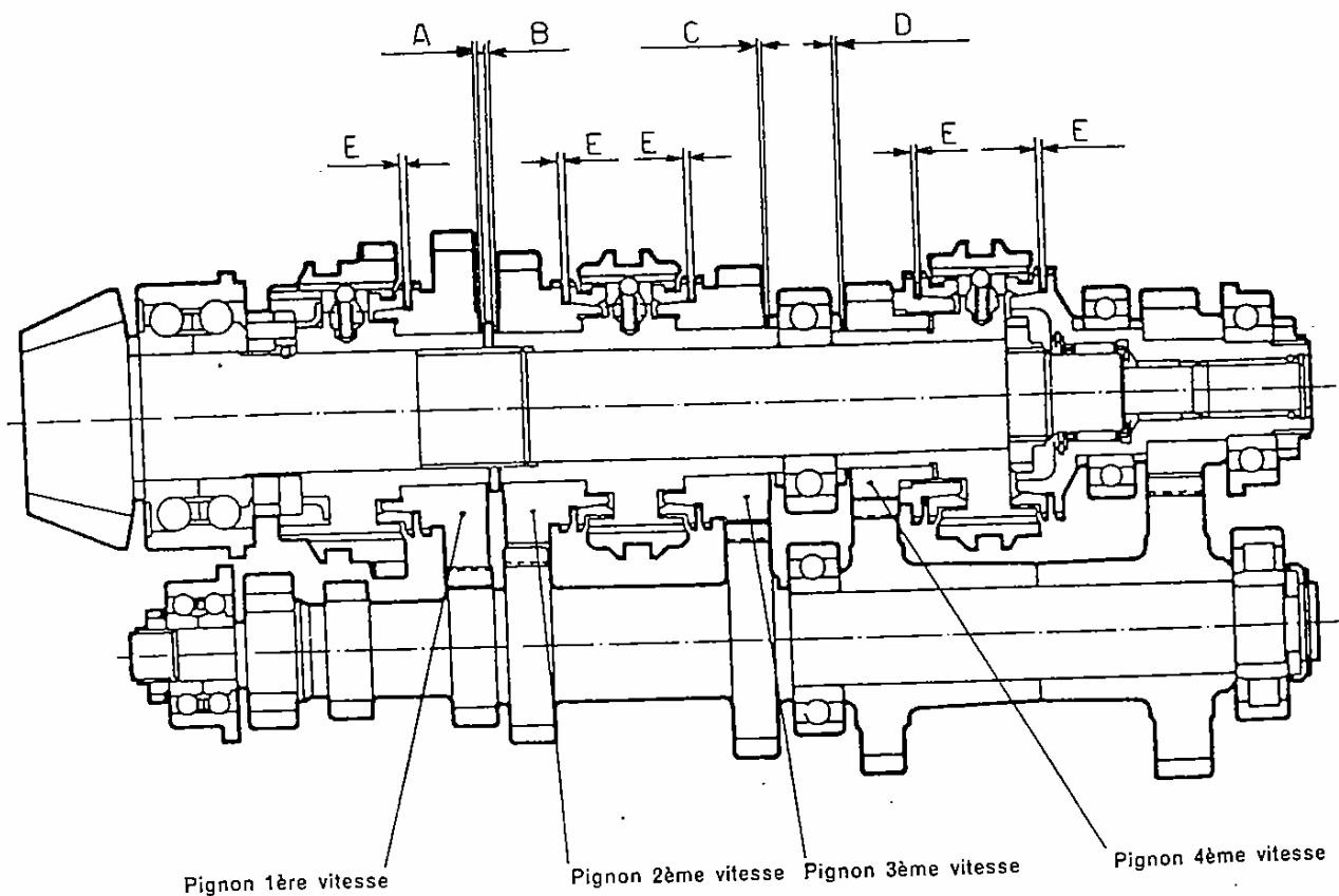
Fig. 16. - Pignonerie boîte à 5 vitesses.
