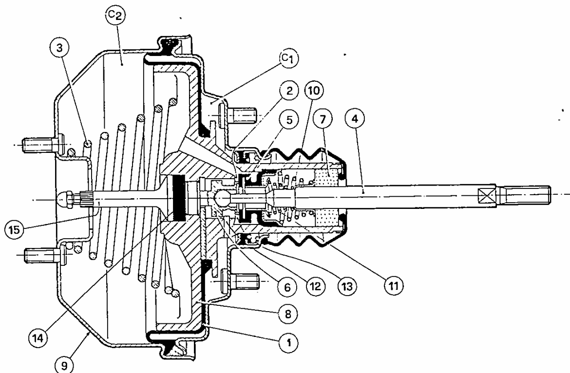
Fig. 26. - Coupe du servo-frein.
