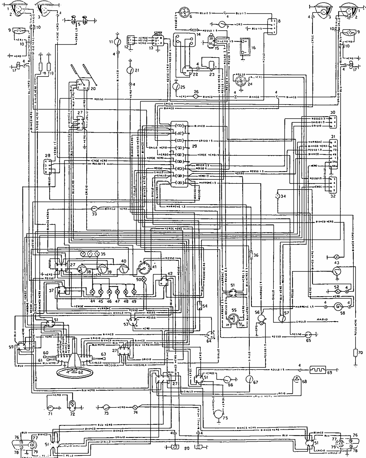
Schéma installation électrique Coupé 1600 HF (818.740).
