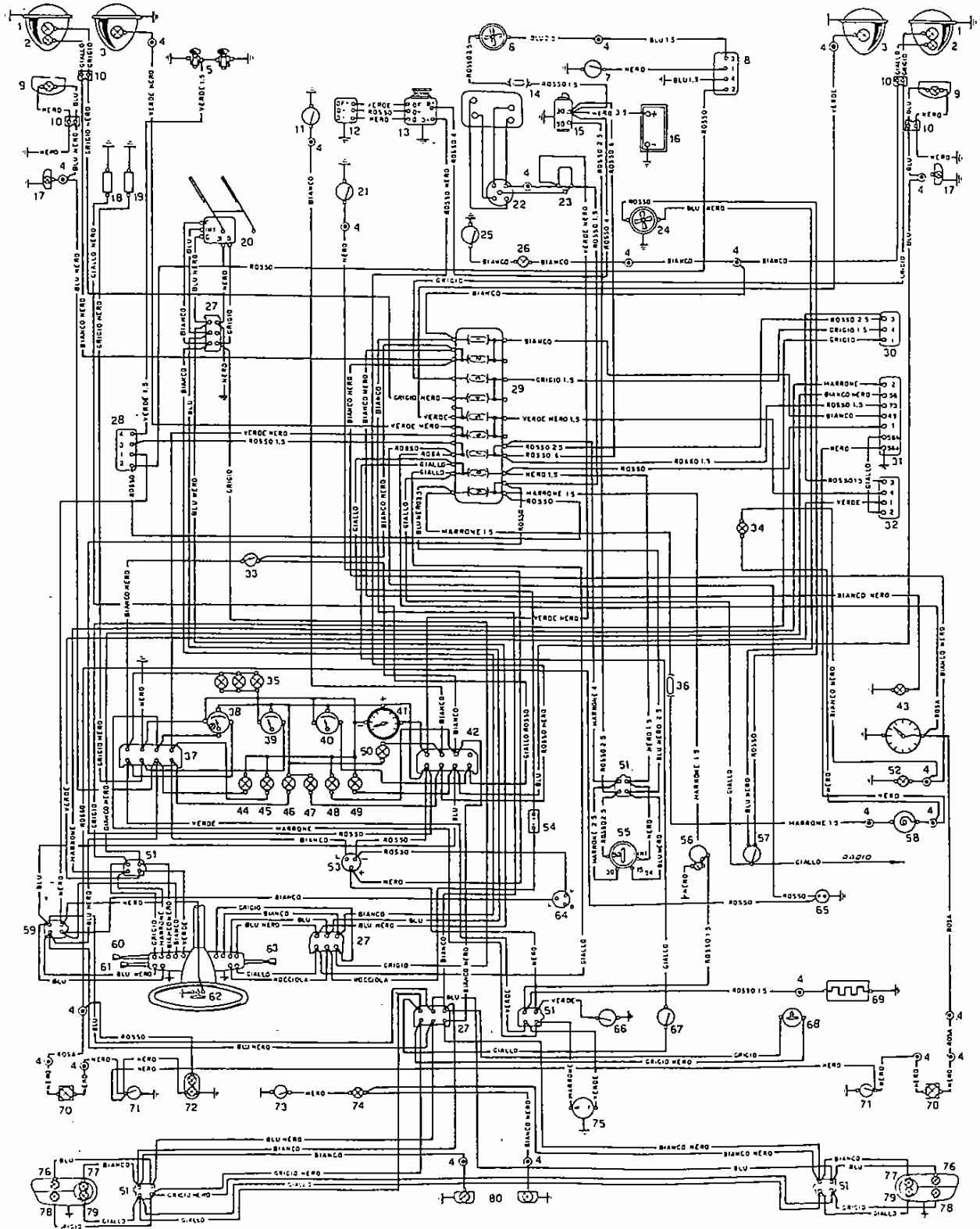
Schéma installation électrique coupé (818.630).
